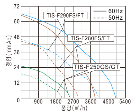
성능곡선
